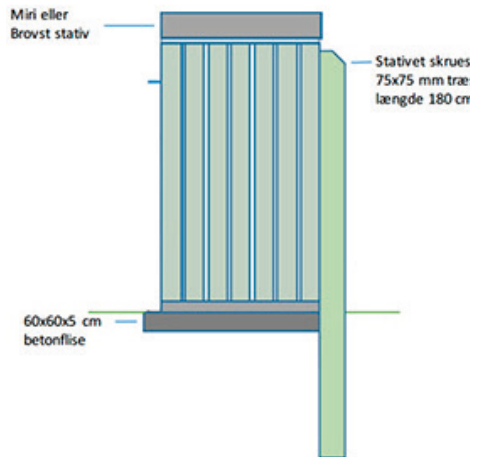
Opstilling af træbeklædt affaldsstativ ved vej
